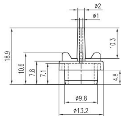
Εικόνα 1: Ακροφύσιο
